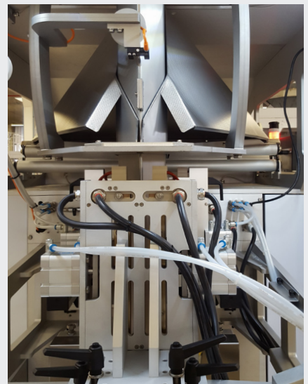
Dettagli del saldante verticale e tubo formatore
