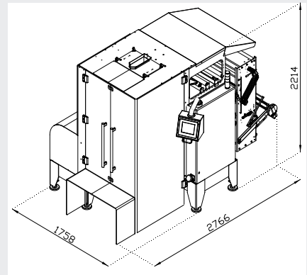
Dimensioni Macchina
